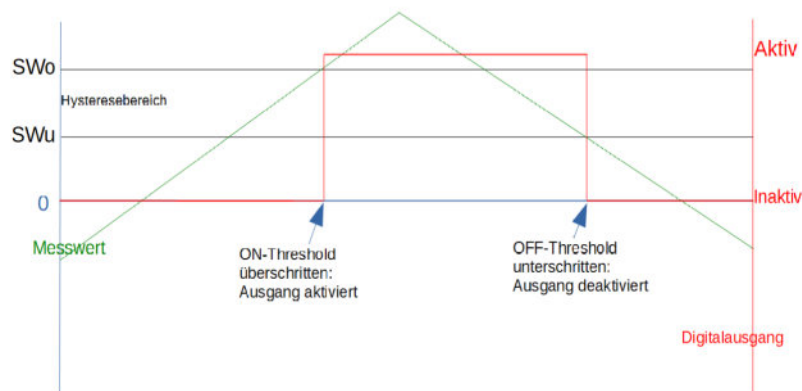
Schwellwertschalter mit Hysteresis
