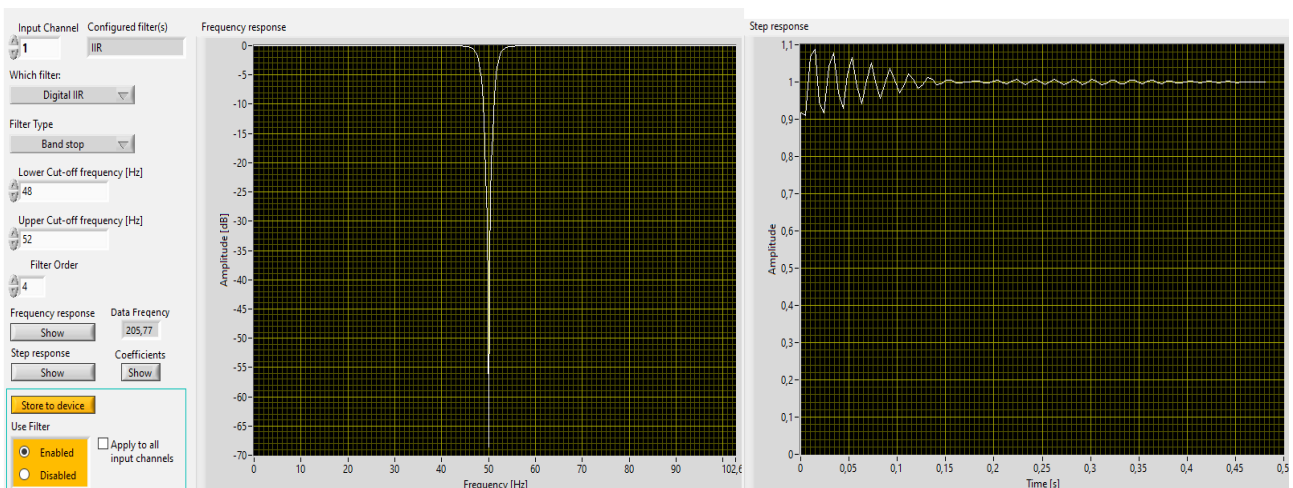
IIR Bandsperre zur Dämpfung von 50 Hz (Netzbrumm).
