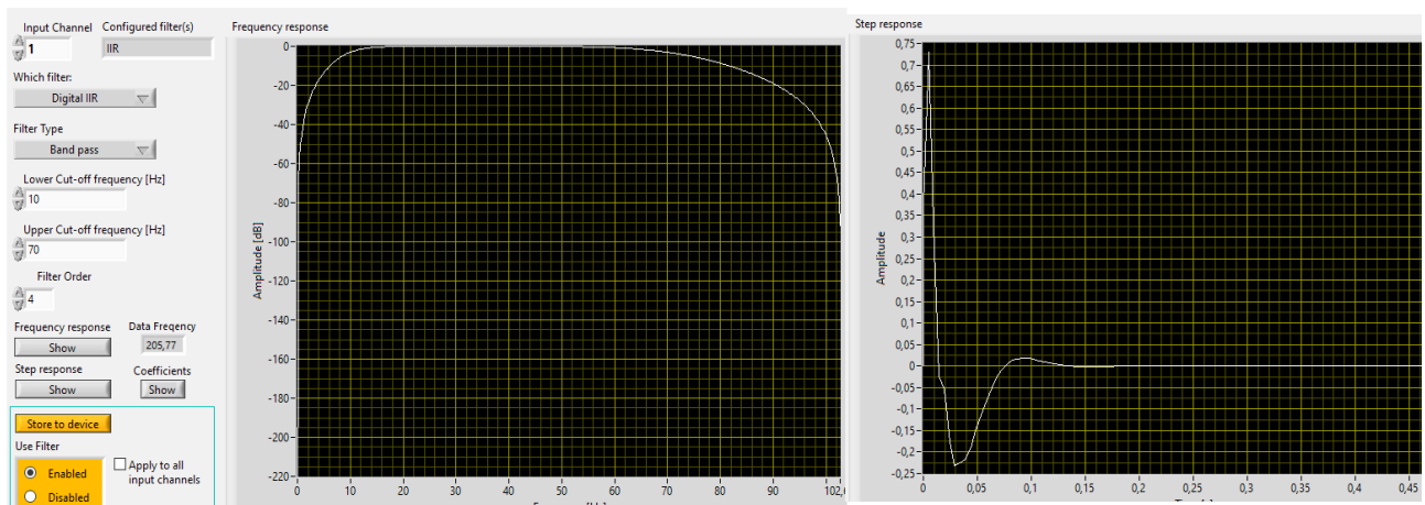
IIR Bandpass von F_a/20 bis F_a \cdot 0,35 . Die Sprungantwort ähnelt der des Hochpasses.
