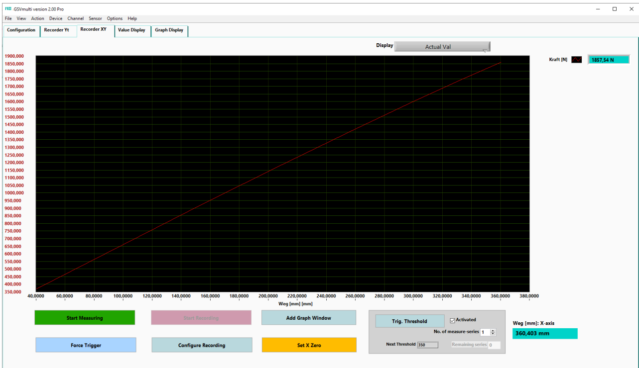
Beispiel: XY Recorder für Kraft-Weg-Messung
