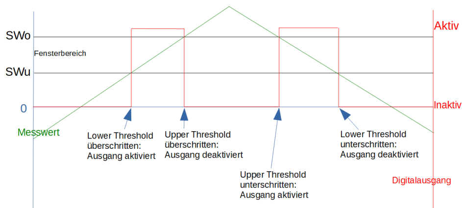
Fensterkomparator
