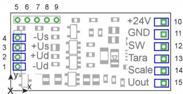
Abbildung 3: Anschlussbelegung, Ansicht: Oberseite
