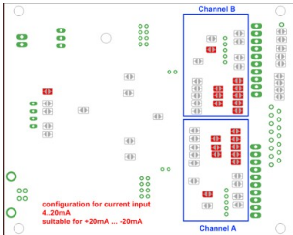
Abbildung 9: Stromeingang 4-20mA
