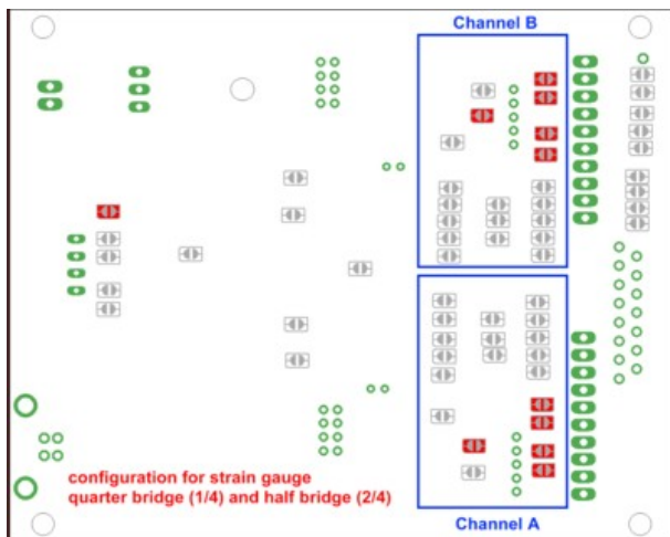
Abbildung 6: DMS Viertelbrücken 350 Ohm und Halbbrücken (120 Ohm...5000 Ohm)
