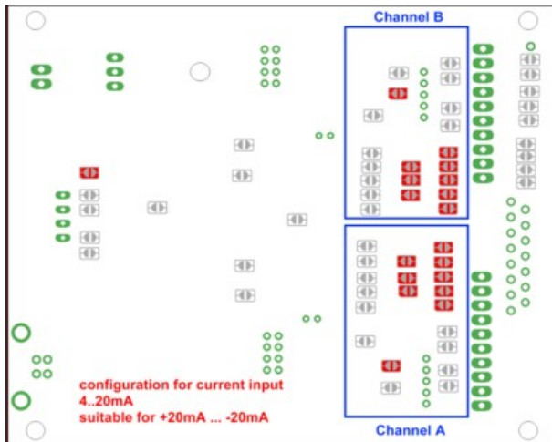
Abbildung 9: Stromeingang 4-20mA
