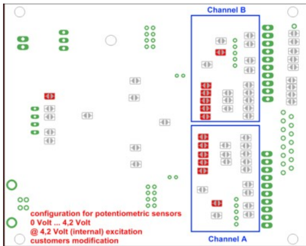
Abbildung 7: Potentiometrische Geber, Wegsensoren
