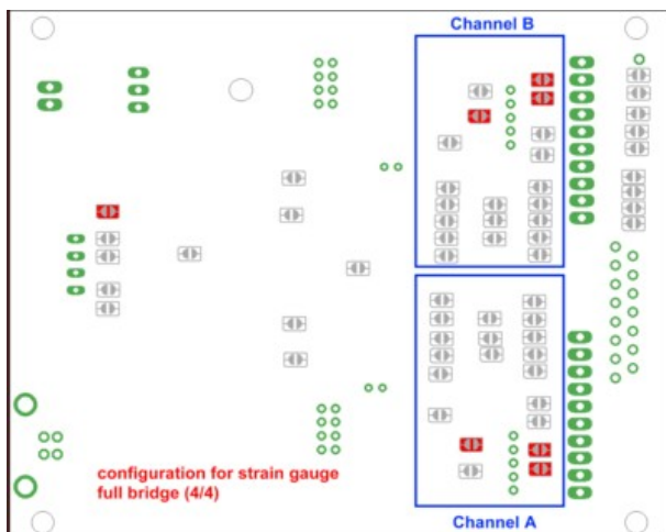
Abbildung 5: DMS Vollbrücken
