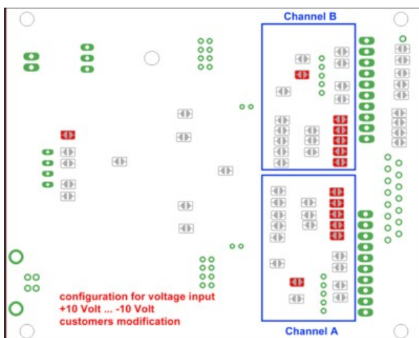
Abbildung 8: Spannungseingang +-10 Volt
