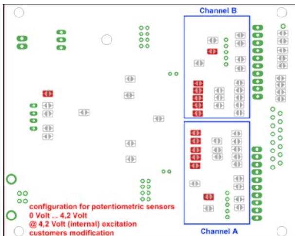
Abbildung 7: Potentiometrische Geber, Wegsensoren
