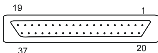
Abbildung 1: 37-pol. Sub-D Buchse
